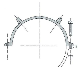
Coupe des segments PA/PE 6 à PA/PE 12, collier avec 6 patins
