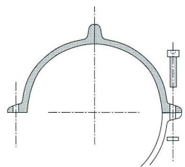
coupe des segments PA/PE 0,75 à PA/PE 4, collier avec 4 patins
